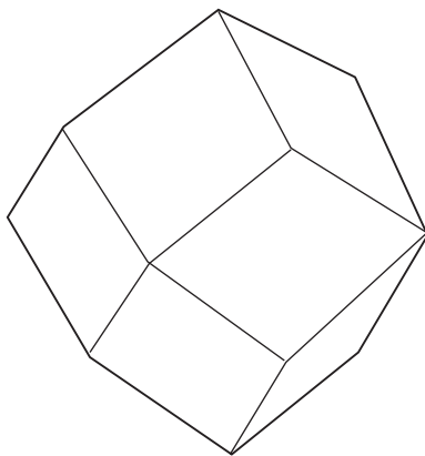
Cubic
