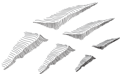
Seif dune
