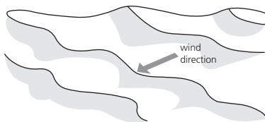
Aklé dune
