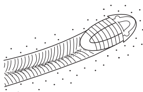
Cruziana
