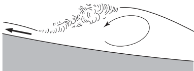
Spilling breaker
