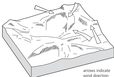
Star dune
