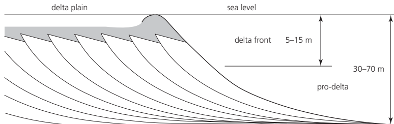
Pro-delta
