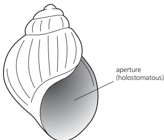
Aperture
