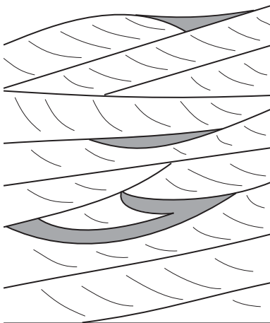
Flaser bedding
