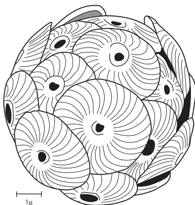
Coccolithophorid
