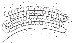
Nereites
